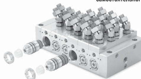
Кассетный монтаж клапанов (в одну кассету устанавливаются два клапана с шагом 30 мм)
