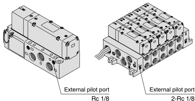
<Sub-plate>
